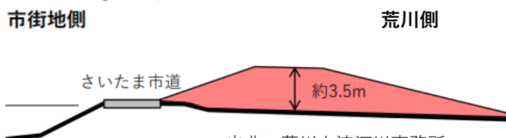
③治水橋の堤防高
